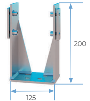
Supporto regolabile
